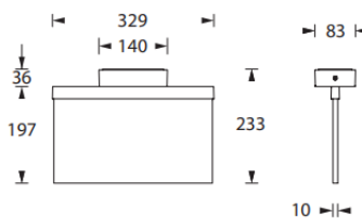
Masse Deckenmontage 329 x 233 x 83mm
