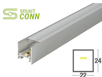
LED-Profil L2422
