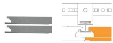
Einbaurahmen Modul 625
