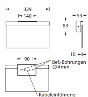
Masse Wandmontage 329 x 203 x 53mm
