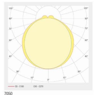
Abstrahlung
