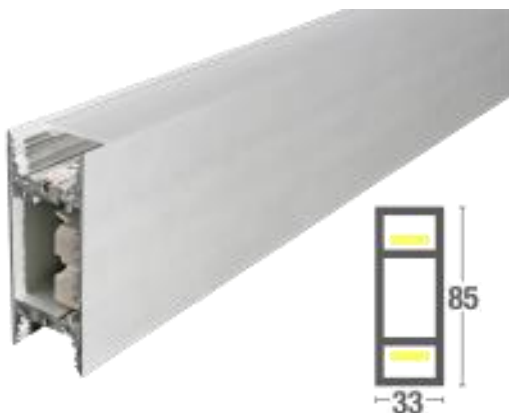
Profil
