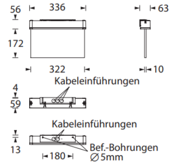
Masse Wandmontage 336 x 228 x 63mm
