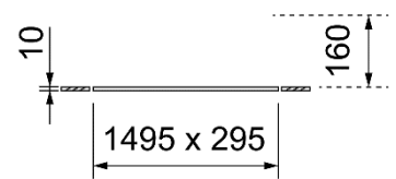
Modul Long 1500 Nicht für Kombination mit Spannfeder-SET geeignet!
