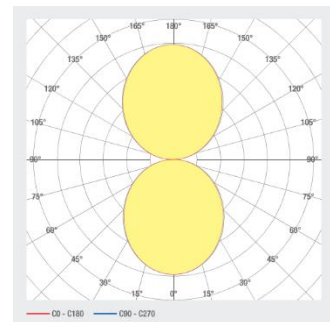
Abstrahlung
