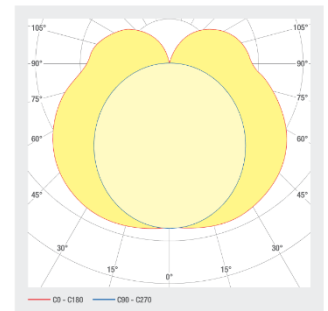
Abstrahlung
