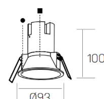
Ausschnitt Ø 85mm
