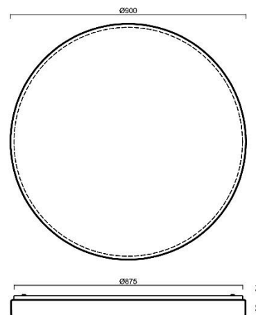
DELIA 5
