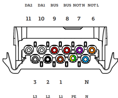
Durchgangsverdrahtung
