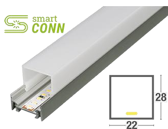
LED-Profil U2822
