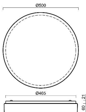
DELIA 3
