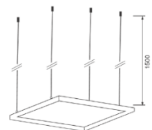
Aufhängung ohne Baldachin
