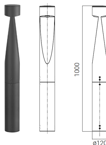
IANUS 1000 double
