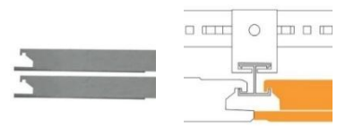
Einbaurahmen Modul 625
