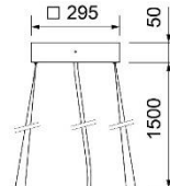
Aufhängung ohne Baldachin
