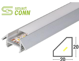
LED-Profil 2020
