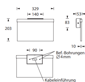
Masse Wandmontage 329 x 203 x 53mm
