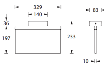
Masse Deckenmontage 329 x 233 x 83mm
