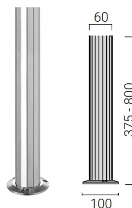
Poller Edelstahl H 375 / 800
