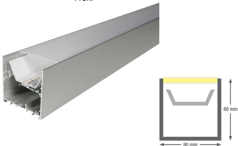
Profil
