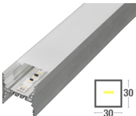
Profil
