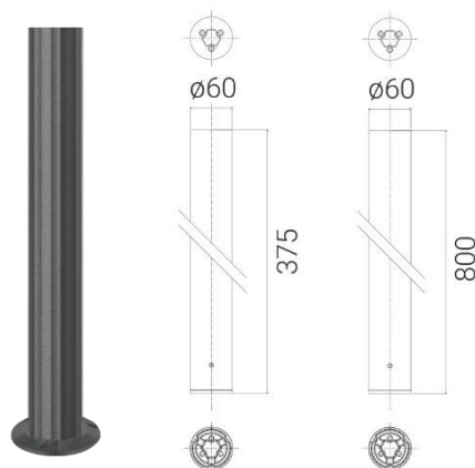
Poller Alu H 375 / 800
