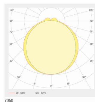
Abstrahlung
