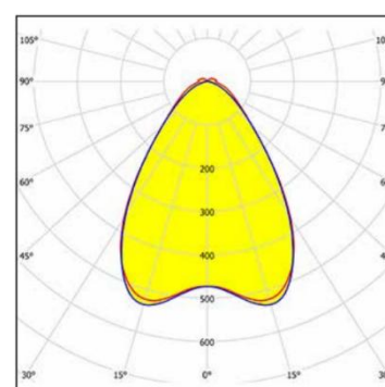
ATEX ROCK MEDIUM (Tief-/Breitstrahlend)
