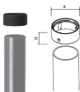
Adapter für alle Masten Ø 60mm
