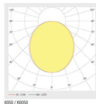
Abstrahlung
