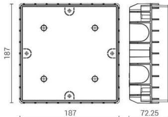
STAMP Einbaugehäuse & Masse
