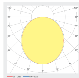
Abstrahlung
