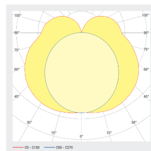
Abstrahlung
