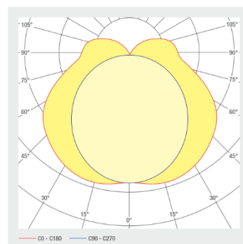
Abstrahlung
