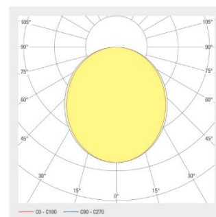
Abstrahlung
