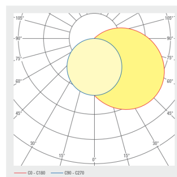
Abstrahlung
