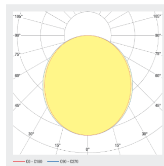
Abstrahlung
