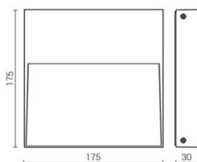
STAMP Einbaugehäuse & Masse
