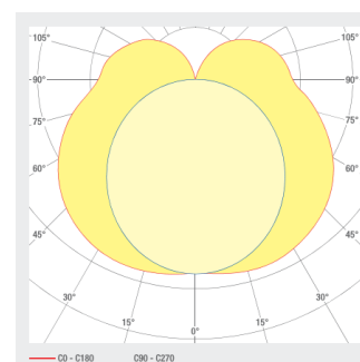
Abstrahlung
