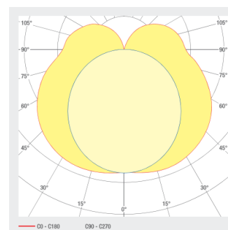
Abstrahlung
