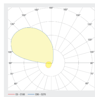
Abstrahlung
