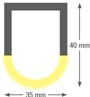
Massbild
