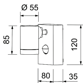
ZAKY II MONO mit PIR
