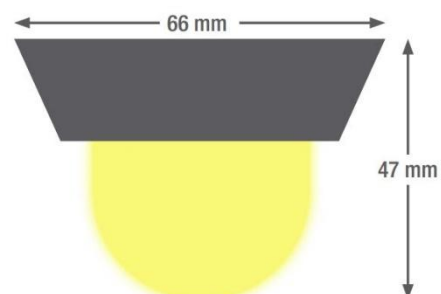
Massbild
